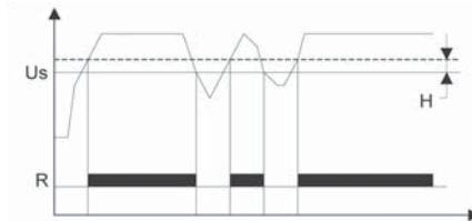
Диаграмма работы E 236-US 1.1 и US 2.1
