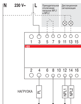
Однофазная схема подключения
