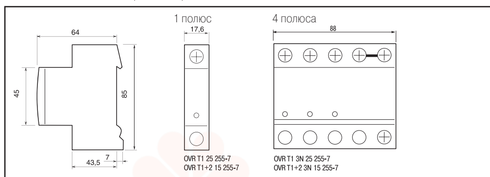
УЗИП Тип 1 и Тип 1+2 ( I_{ff} = 7 \text{ кА} )
