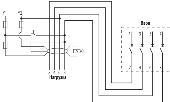
DDA 204 AE
