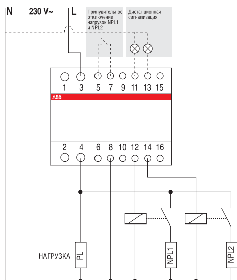
Однофазная схема подключения неприоритетных нагрузок с номинальным током более 16А
