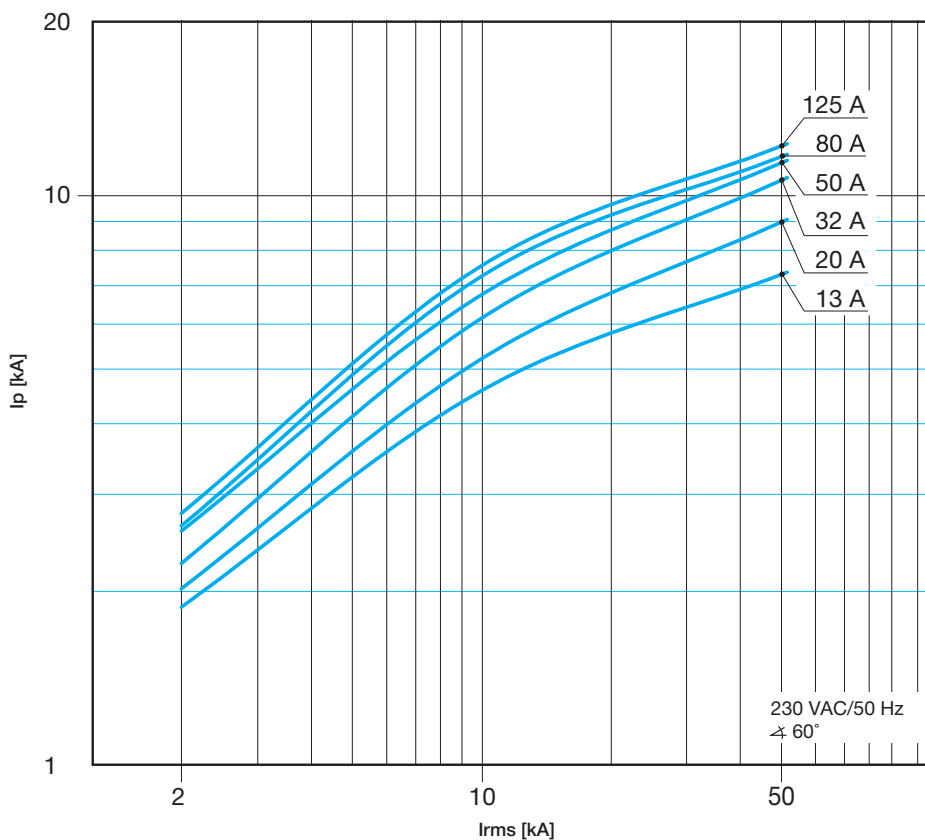
S 800 S характеристики В, С, D и К
