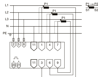
- Косвенное подключение (через ТТ)
