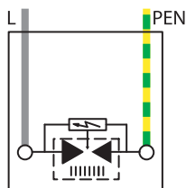
OVR T1 25 440-50
