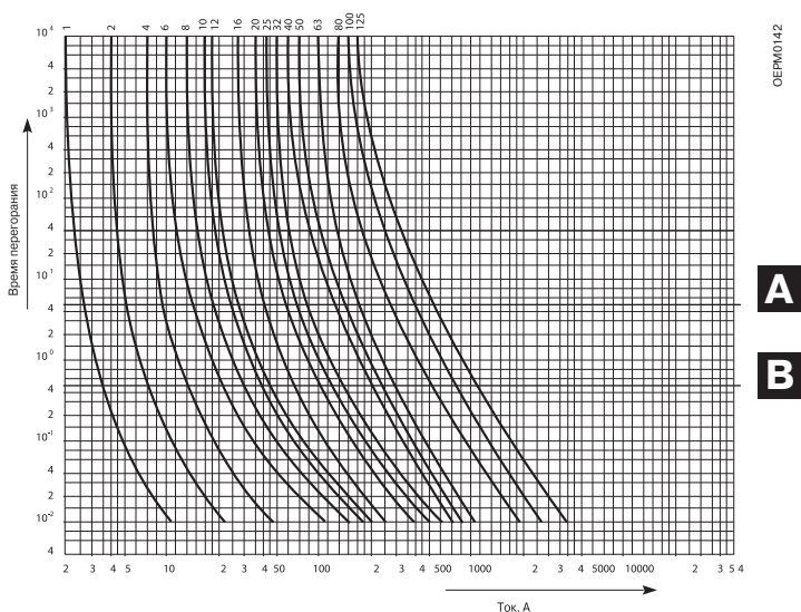
Цилиндрические предохранители типа aM
