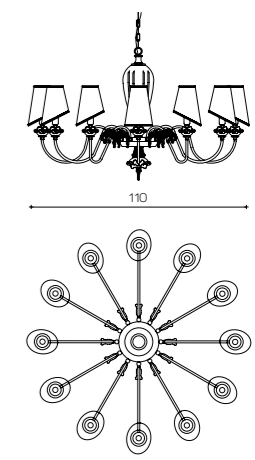
Art. 1774/CH12 ø 110 cm H 66 cm Pø 14 cm 12 x E14 x 40W
