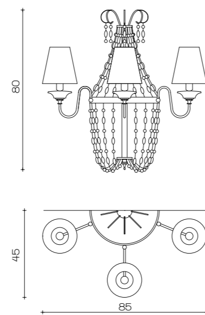
Art. 1380/A3 ø 85 cm H 80 cm Pø 18 cm 3 x E14 x 40W
