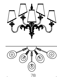
Art.1774/A5 H 56 cm ø 78 cm Sp 42 cm Pø 14 cm 5 x E14 x 40W
