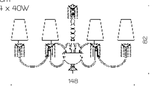
Art. 1508/CH12 ø 190 cm H 120 cm Pø 20 cm 12 x E14 x 40W
