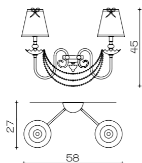
Art. 1794/A2 L 58cm H 45 cm Sp 27 cm Pø 16 cm 2 x E14 x 40W
