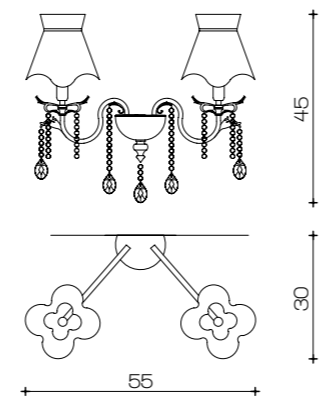
Art. 1689/A2 L 55 cm H 45 cm Sp 30 cm Pø 18 cm 2 x E14 x 40W
