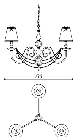
Art. 1794/CH3 ø 78 cm H 45 cm Pø 16 cm 3 x E14 x 40W
