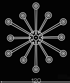
Art. 1761/CH12 ø 120 cm H 150 cm Pø 16 cm 12 x E14 x 40W
