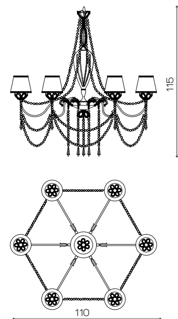
Art. 1744/CH6/ORO24K ø 110 cm H 115 cm Pø 16 cm 6 x E14 x 40W
