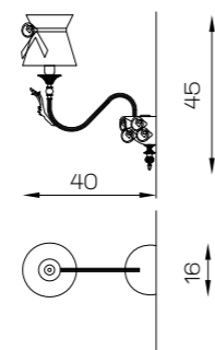
Art. 1850/A1 Pø 16 cm H 45 cm Sp 40 cm 1 x E14 x 40W
