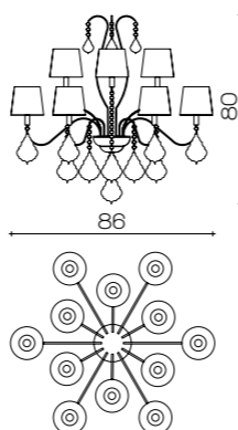
Art. 1742/CH12/KR/V2 ø 86 cm H 80 cm Pø 14 cm 8 x E14 x 25W
