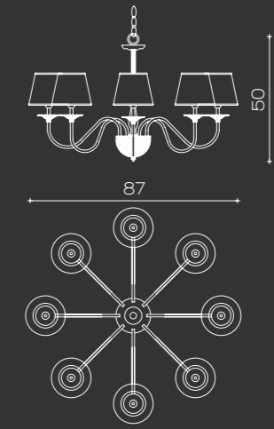
Art. 1460/CH8 ø 87 cm H 50 cm Pø 16 cm 8 x E14 x 40W
