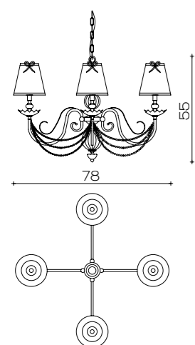
Art. 1794/CH4 ø 78 cm H 55 cm Pø 16 cm 4 x E14 x 40W
