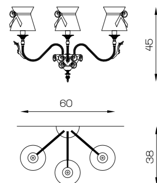
Art. 1850/A3 L 60 cm H 45 cm Sp 38 cm 3 x E14 x 40W
