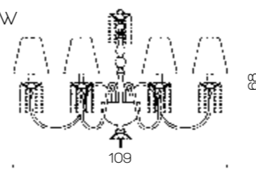
Art. 1507/CH8 ø 148 cm H 82 cm Pø 18 cm 8 x E14 x 40W
