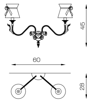
Art. 1850/A2 L 60 cm H 45 cm Sp 28 cm 2 x E14 x 40W
