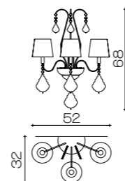
Art. 1742/A3/KR ø 52 cm H 68 cm Pø 14 cm 3 x E14 x 25W
