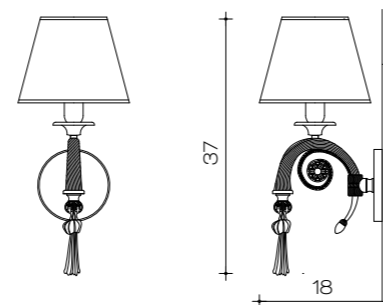
Art. 1162/A Pø 18 cm H 37 cm Sp 18 cm 1 x E14 x 40W
