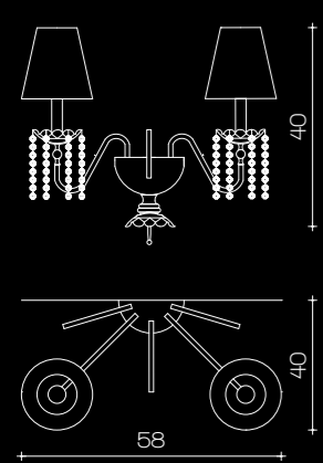
Art. 1451/A2 KR ø 58 cm H 40 cm Sp 30 cm Pø 16 cm 2 x E14 x 40W
