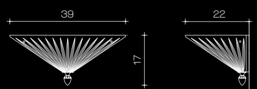
Art.1621/B Applique ø 39 cm H 17 cm 1 x G9 x 40W
