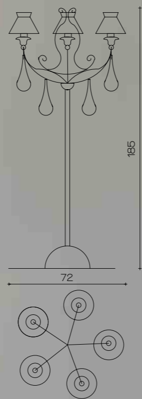
Art. 1823/FL ø 72 cm H180 cm Pø 20 cm 5 x E14 x 40W
