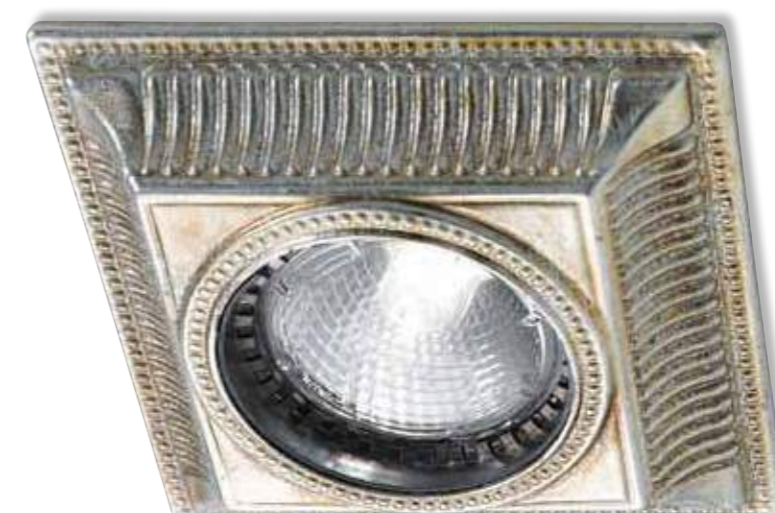
14305/F6 Ø 10x10 cm - sp. 2 cm - 1 x GZ10 50W max
