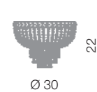
Settat plafoniera Ø 30 cm Ø 30 cm - H 22 cm 3 x E14 40W
