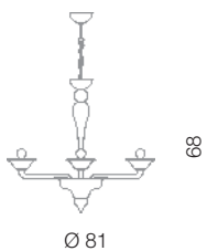
Ca' d'Oro lampadario 3L Ø 81 cm - H 68 cm 3 x E14 40W
