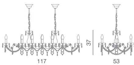
Graz lampadario 12L L 117 cm - H 37 cm - SP 53 cm 12 x E14 40W
