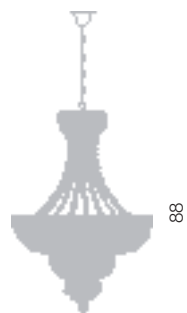
Beethoven lampadario Impero Ø 60 cm Ø 61 cm - H 88 cm 9 x E14 40W
