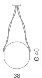
Golf sospensione Ø 40 cm L 38 cm - Ø 40 cm - H max 120 cm 2 x E27 75W
