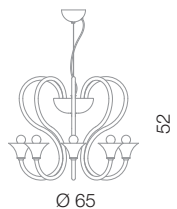
Babylon lampadario 8L Ø 65 cm - H 52 cm 8 x E14 40W
