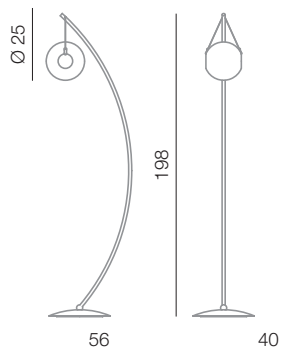
Golf terra 1L L 56 x 40 cm - Ø 25 cm - H 198 cm 1 x E27 75W
