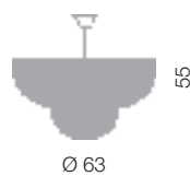
Amsterdam sospensione Ø 60 cm Ø 63 cm - H 55 cm 8 x E14 40W
