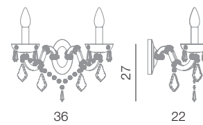
Graz parete 2L L 36 cm - H 27 cm - SP 22 cm 2 x E14 40W
