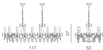
Graz lampadario 16L L 117 cm - H 37 cm - SP 53 cm 16 x E14 40W
