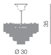
Mosca sospensione Ø 30 cm Ø 30 cm - H 35 cm 3 x E14 40W
