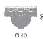
Pegaso plafoniera Ø 40 cm Ø 40 cm - H 30 cm 4 x E14 40W
