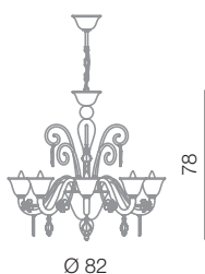
Alvisse lampadario 8L Ø 82 cm - H 78 cm 8 x E14 40W
