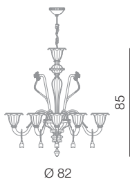
Doge lampadario 8L Ø 82 cm - H 85 cm 8 x E14 40W
