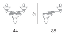
Ca' d'Oro parete 2L L 44 cm - H 31 cm - SP 38 cm 2 x E14 40W
