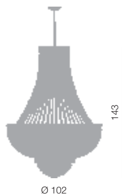
Amsterdam lampadario Impero Ø 100 cm Ø 102 cm - H 143 cm 18 x E14 40W
