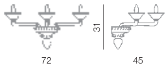
Ca' d'Oro parete 3L L 72 cm - H 31 cm - SP 45 cm 3 x E14 40W
