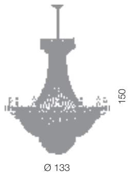
Pegaso lampadario Impero Ø 100 cm Ø 133 cm - H 150 cm 28 x E14 40W
