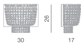
Amsterdam parete 3L L 30 cm - H 26 cm - SP 17 cm 3 x E14 40W
