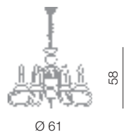
Miró lampadario 6L Ø 61 cm - H 58 cm 6 x E14 40W
