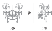
Erika parete 2L L 38 cm - H 36 cm - SP 26 cm 2 x E14 40W
