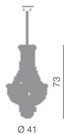
Osaka lampadario Impero Ø 40 cm Ø 41 cm - H 73 cm 6 x E14 40W
