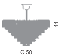
Mosca sospensione Ø 50 cm Ø 50 cm - H 44 cm 4 x E14 40W
