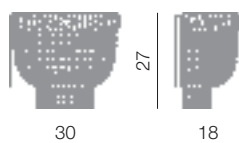
Roma parete 3L L 30 cm - H 27 cm - SP 18 cm 3 x E14 40W
