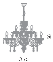
Toledo lampadario 8+4L Ø 75 cm - H 58 cm 12 x E14 40W
