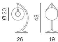
Golf tavolo 1L L 26 x 19 cm - Ø 20 cm - H 48 cm 1 x E27 60W
