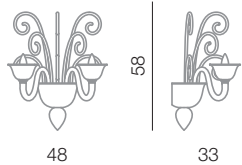
Barnaba parete 2L L 48 cm - H 58 cm - SP 33 cm 2 x E14 40W
