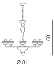
Ca' d'Oro lampadario 8L Ø 81 cm - H 68 cm 8 x E14 40W
