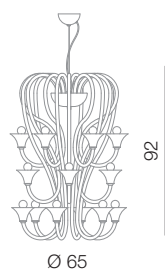
Babylon lampadario 18L (6+6+6) Ø 65 cm - H 92 cm 18 x E14 40W
