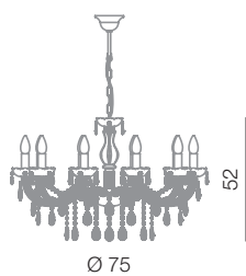
Vienna Plus lampadario 10L Ø 75 cm - H 52 cm 10 x E14 40W
