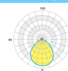
КСС ТИП «Д»
