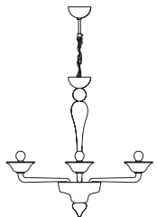
Ca' d'Oro lampadario 3L Ø 81 cm - H 68 cm 3 x E14 40W
