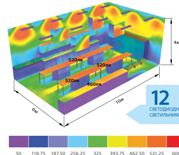
Светодиодные светильники «ТИТАН»
