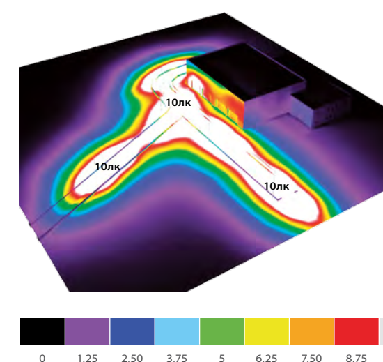
Светодиодные светильники «КЕДР 75»
