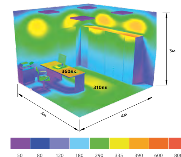
Светодиодные светильники «ОФИС»
