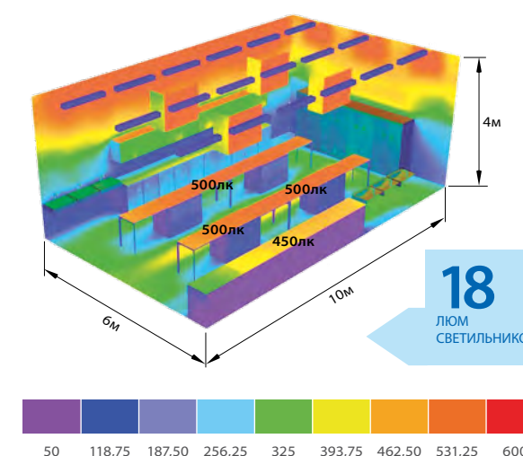
Люминесцентные светильники «ЛСП 2x36»
