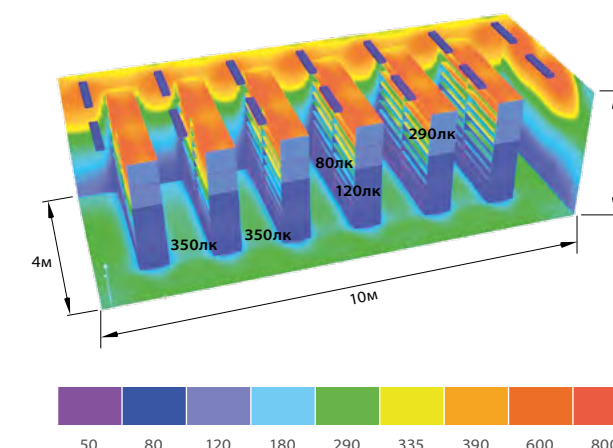
Светодиодные светильники «ТИТАН»
