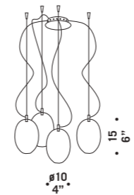
PRO•SECCO S4D 4x20W-12V G4 HSGST/UB alogeno bispina halogen bi-pin cavo elettrico 200 cm trasformatore elettronico cables lenght 200 cm electronic transformer
