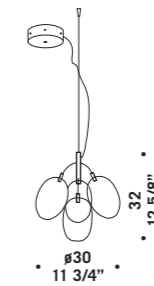
PRO•SECCO S4DG 4x20W-12V G4 HSGST/UB alogeno bispina halogen bi-pin cavo elettrico 200 cm trasformatore elettronico cables lenght 200 cm electronic transformer
