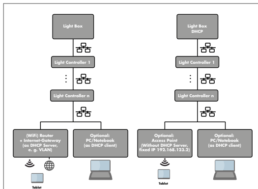
Архитектура системы
