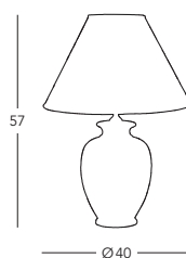
■ 0014.74.3 Tischleuchte/table lamp 💡 1 lp., E27, 100 W
