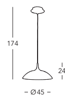
A1304.31.6.W/45 Hängeleuchte/hanging lamp 1 Ip., E27, 100 W
