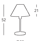
264.70.4 Tischleuchte/ table lamp 1 Ip., E27, 60 W
