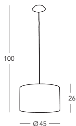
A1307.33R.6 Hängeleuchte/hanging lamp 3 lp., E27, 60 W inkl. Lichtblende/ incl. light diffuser
