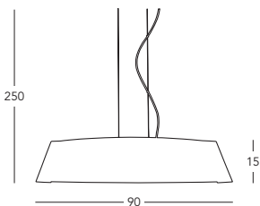
2295.31L.3.W Hängeleuchte / hanging lamp 1 Ip., LED, 13 W 940 Lumen, 2900 Kelvin
