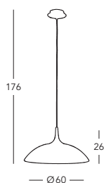
A1304.31.6.Cu/60 Hängeleuchte/hanging lamp 💡 1 lp., E27, 100 W
