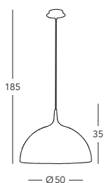
■ A1305.31.7.W/50 Hängeleuchte / hanging lamp 💡 1 lp., E27, 100 W
