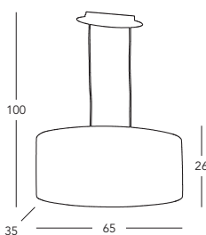
■ A1307.33O.7 Hängeleuchte / hanging lamp ☏ 3 lp., E27, 60 W inkl. Lichtblende / incl. light diffuser
