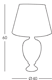
0094.70 Tischleuchte / table lamp ☑ 1 lp., E27, 100 W
