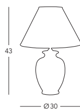
0014.70 Tischleuchte / table lamp 1 Ip., E27, 100 W
