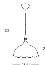
731.30.125 Hängeleuchte/hanging lamp 1 Ip., E27, 75 W
