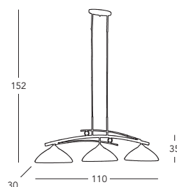
■ 253.83.7.W Balken / chandelier ☑ 3 lp., E27, 75 W
