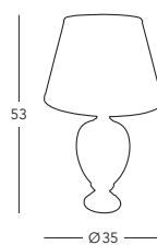
780.70 Tischleuchte / table lamp ☑ 1 lp., E27, 60 W
