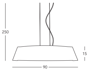
■ 2295.31L.3.Au Hängeleuchte / hanging lamp 💡 1 Ip., LED, 13 W 940 Lumen, 2900 Kelvin
