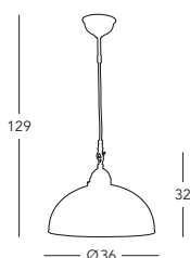
731.32.129 Hängeleuchte/hanging lamp 1 Ip., E27, 75 W
