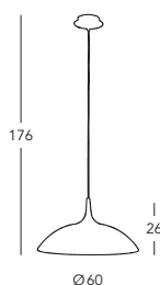
A1304.31.7.W/60 Hängeleuchte/hanging lamp 1 Ip., E27, 100 W
