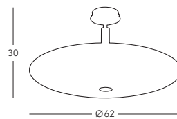
0296.55L.5.WW abgehängte Deckenleuchte/ suspended ceiling lamp 5 Ip., E14, 60 W verchromt/ chrome plated
