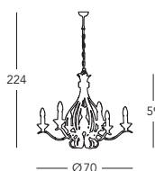
0144.86 Luster / chandelier ☑ 6 lp., E14, 60 W
