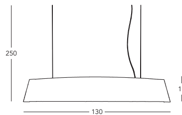
■ 2295.32.3.Au Hängeleuchte / hanging lamp 💡 2 Ip., LED, 13 W 1880 Lumen, 2900 Kelvin ohne Abbildung / without illustration
