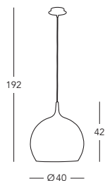
A1306.31.7.Cu/40 Hängeleuchte / hanging lamp 1 Ip., E27, 100 W
