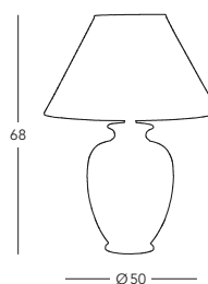
■ 0014.75 Tischleuchte/table lamp ☹ 1 lp., E27, 100 W
