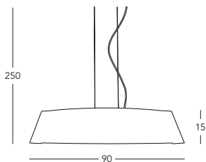
2295.31L.5.W Hängeleuchte / hanging lamp 1 Ip., LED, 13 W 940 Lumen, 2900 Kelvin
