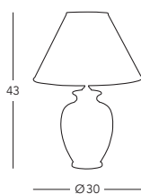
■ 0014.73.3 Tischleuchte/table lamp 💡 1 lp., E27, 100 W
