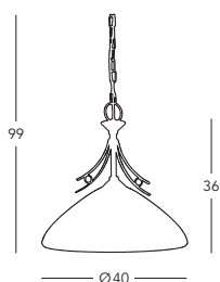
■ 253.31.7.W Hängeleuchte/hanging lamp ☐ 1 Ip., E27, 100 W
