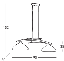
■ 253.82.7.W Balken / chandelier ☑ 2 lp., E27, 75 W
