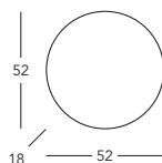
320.13.A Deckenleuchte/ ceiling lamp 3 Ip., E27, 60 W
