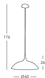
A1304.31.7.Cu/60 Hängeleuchte/hanging lamp 1 Ip., E27, 100 W
