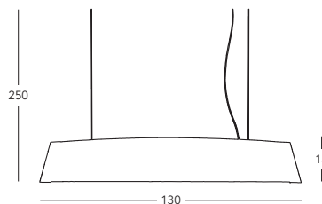
2295.32.3.W Hängeleuchte / hanging lamp 2 Ip., LED, 13 W 1880 Lumen, 2900 Kelvin ohne Abbildung / without illustration
