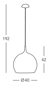
A1306.31.7.Au/40 Hängeleuchte / hanging lamp 1 Ip., E27, 100 W
