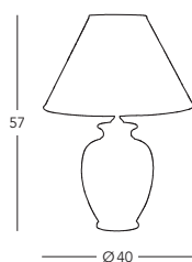
■ 0014.74 Tischleuchte/table lamp ☹ 1 lp., E27, 100 W
