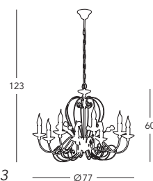
0235.88.YG.KoT Luster/chandelier 8 Ip., E14, 40 W
