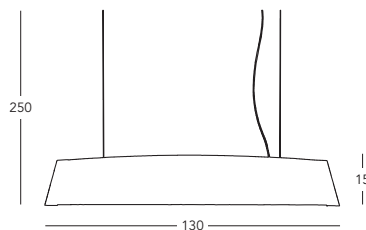
2295.32.5.W Hängeleuchte / hanging lamp 2 Ip., LED, 13 W 1880 Lumen, 2900 Kelvin ohne Abbildung / without illustration
