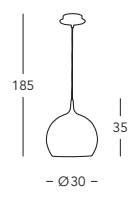
A1306.31.7.Au/30 Hängeleuchte / hanging lamp 1 Ip., E27, 100 W
