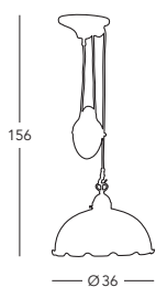
731.33.18 Zughängeleuchte/ hanging lamp ☑ 1 lp., E27, 75 W
