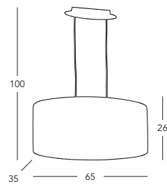
A1307.33O.6 Hängeleuchte/hanging lamp 3 lp., E27, 60 W inkl. Lichtblende/ incl. light diffuser
