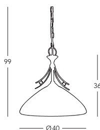
■ 253.31.7.100 Hängeleuchte/hanging lamp ☐ 1 Ip., E27, 100 W
