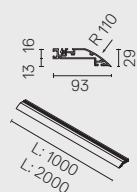
Perfil de Aluminio Aluminium Profile
